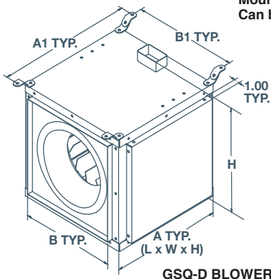
GSQ-D BLOWER
