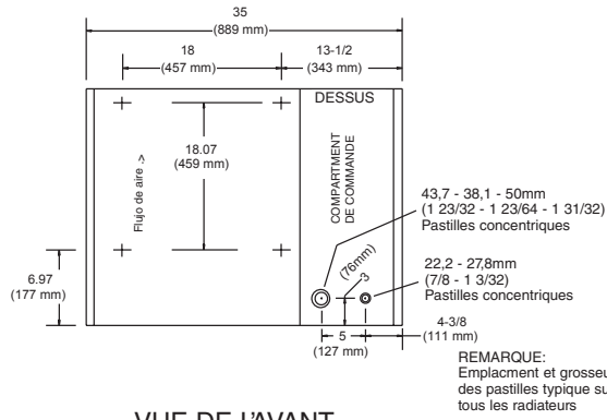
VUE DE L'AVANT 35 po (889 mm)
